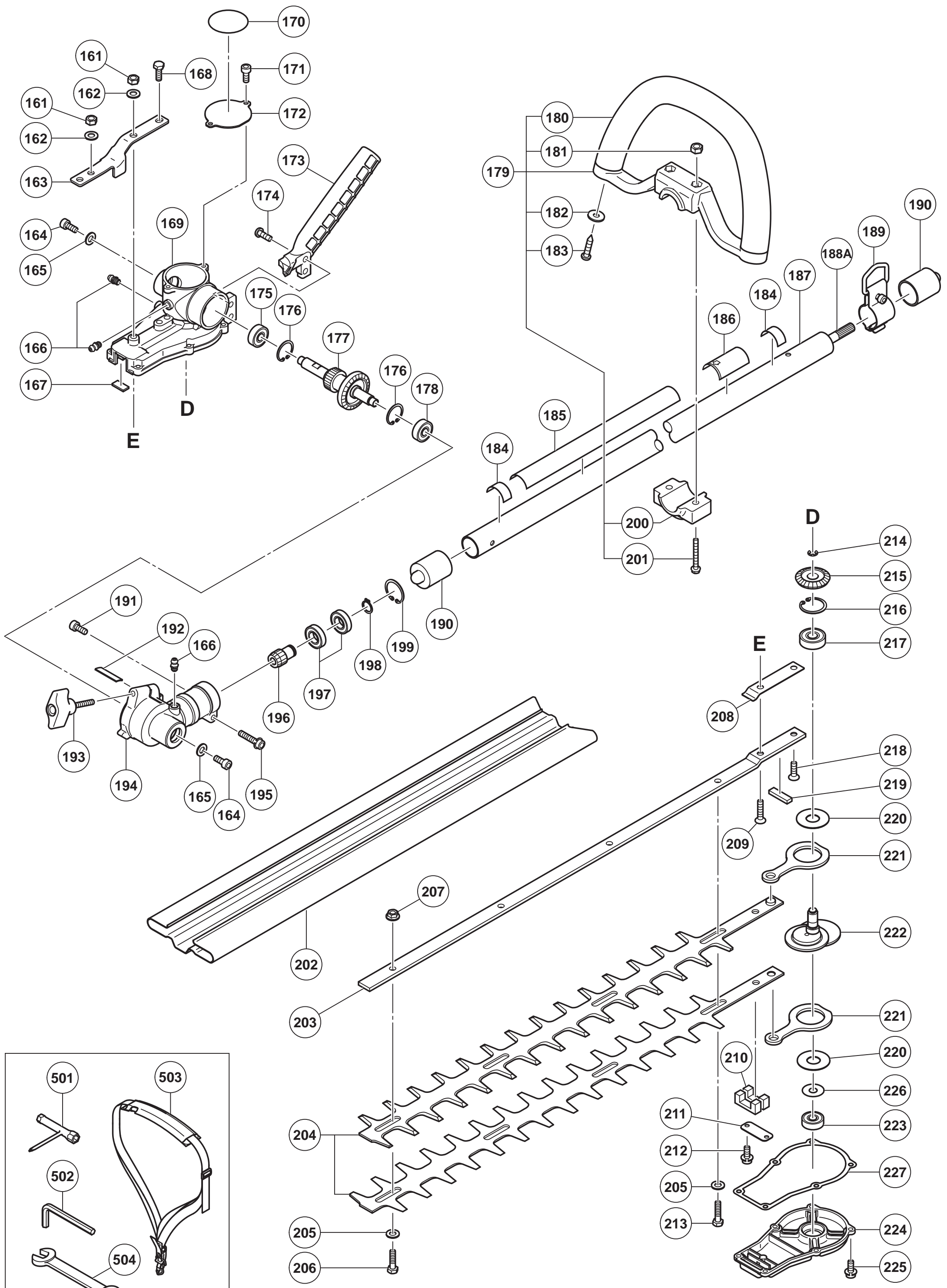
形名 CH27EPAP(3/3)
