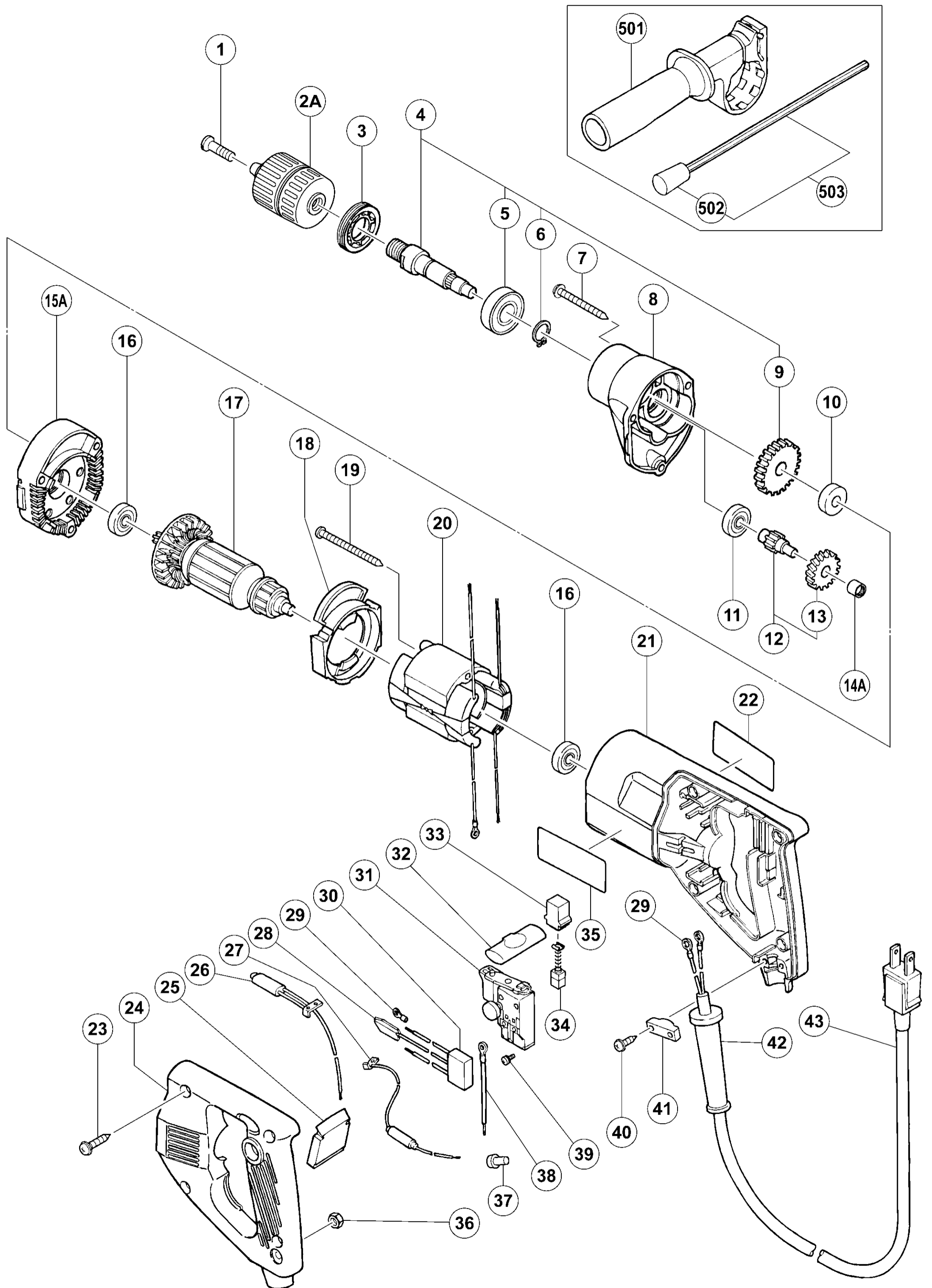
形名 D10SD
