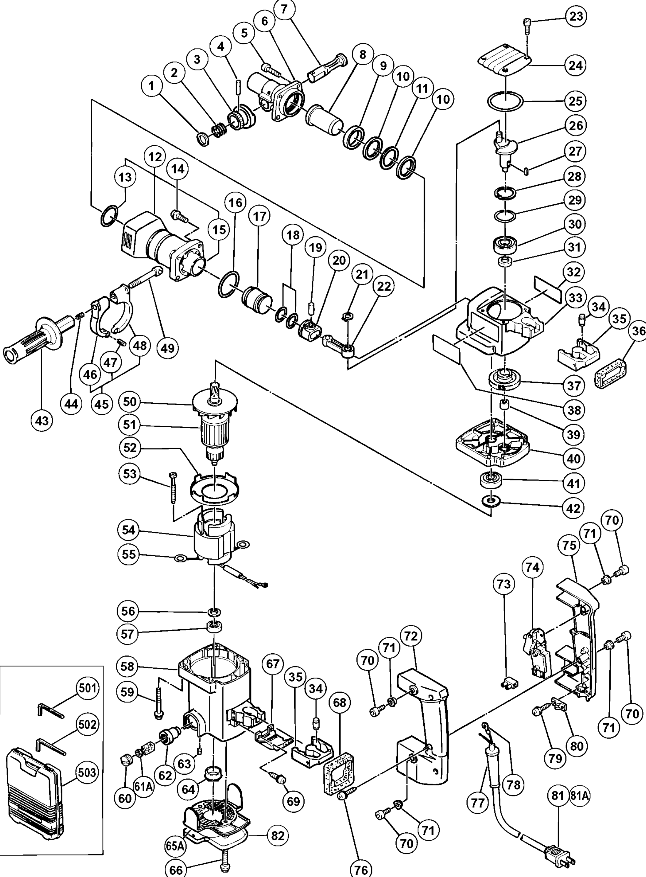
形 名 H45SB2
