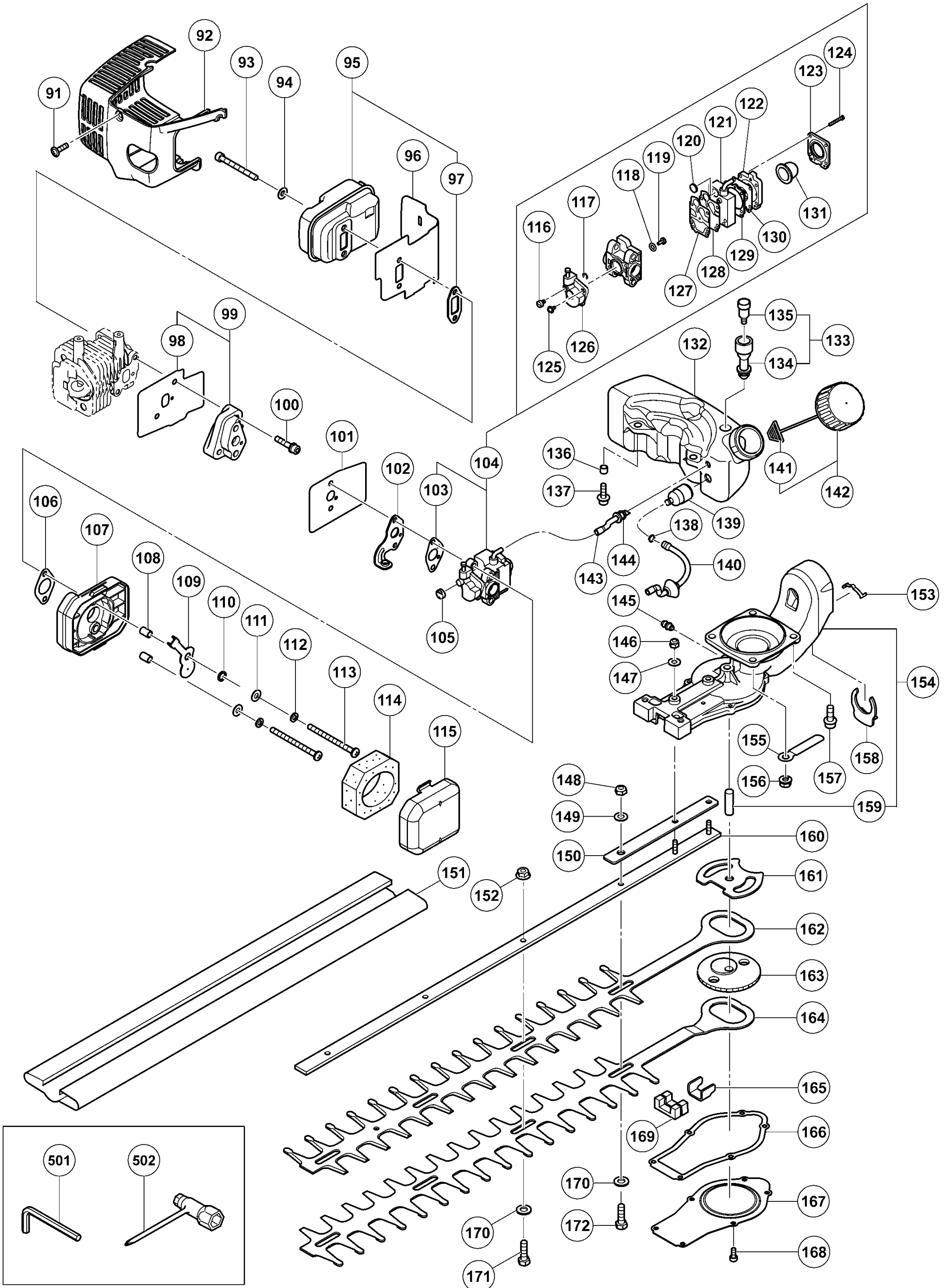
形名 THT-2000SB(2/2)
